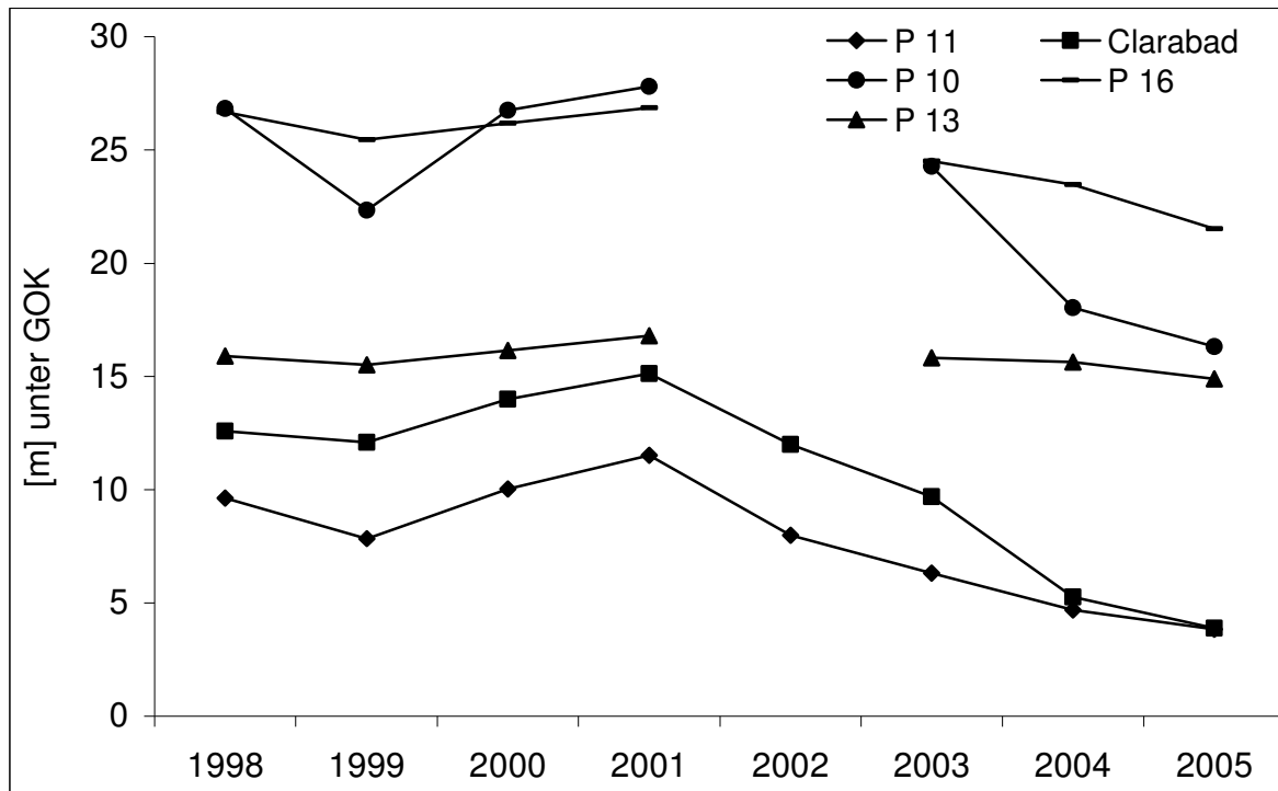
Abbildung 2/10: Durchschnittlicher Wasserstand ausgewählter Grundwassermessstellen im Lappwald in m unterhalb der Geländeoberkante
